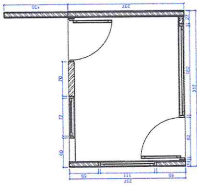
DENAH rencana
